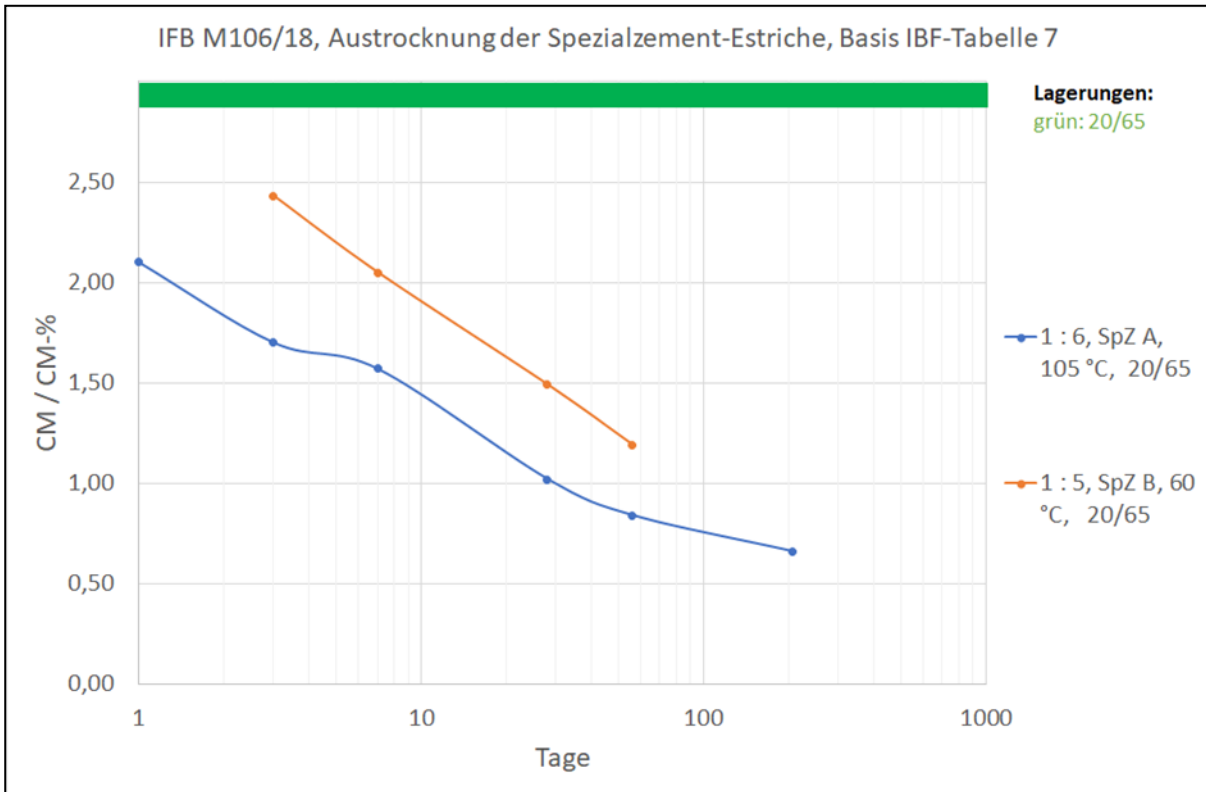
Trocknungskurve der Estriche mit Spezialzement in CM-Werten
