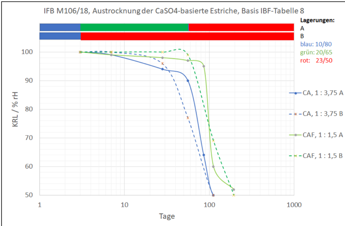
Trocknung der calciumsulfatbasierten Estriche, Zeitachse logarithmisch skaliert
